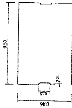
รูปแผ่นฝาปิดรางระบายน้ำ คลส.
