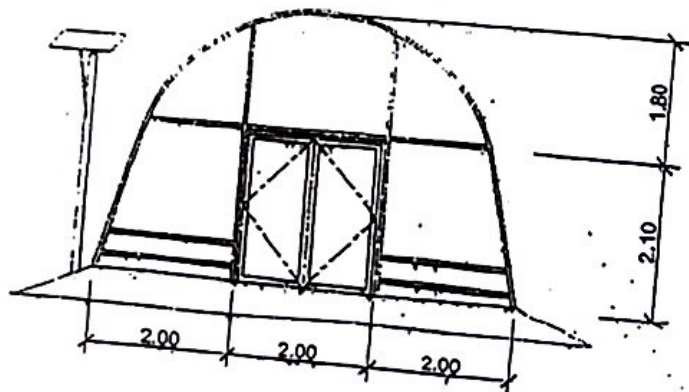
รูปด้านหน้า มาตราส่วน 1:75
